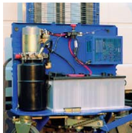
Gut zugänglich sind Pumpe, Batterie, Ladegerät und Elektrik angeordnet.
