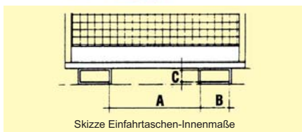
Skizze Einfahrtaschen-Innenmaße
